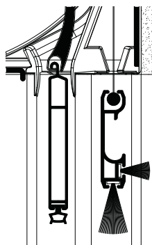
Standard-Bürstenposition in der ISG-Aluminium-Endleiste
