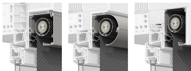
Aluminium-Führung 33 x 96 mm (Flächenbündige FS bei 96 mm Kastentiefe)
