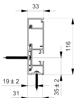
Aluminium-Zusatzprofil für FS 30 x 10 mm, 30 x 20 mm, 30 x 40 mm
