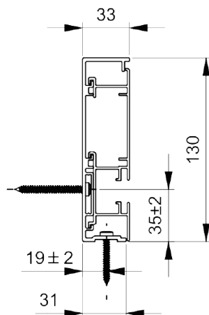
FS Verschlussplatte bis 10° Schräge
