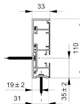
Aluminium-Führung 33 x 110 mm (Flächenbündige FS bei 110 mm Kastentiefe)
